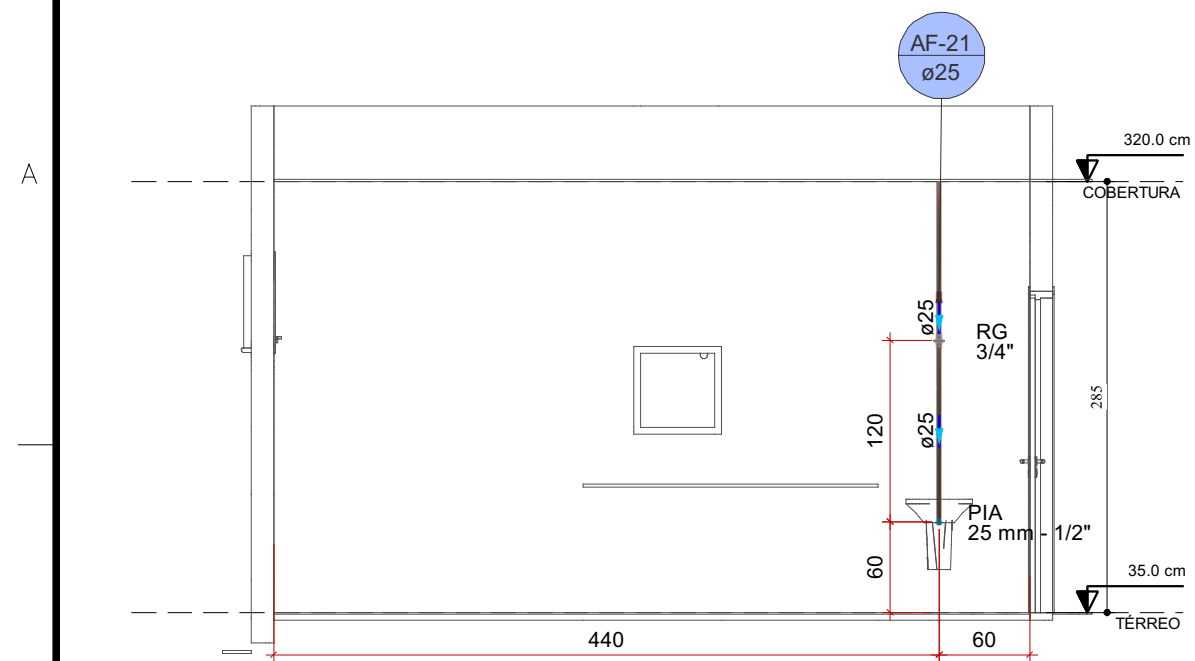
Detalhe HID-20 Escala 1:50
