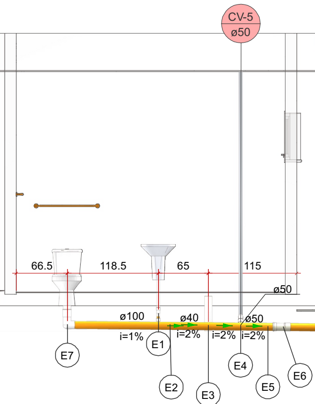
Detalhe SAN-11 Escala 1:50
