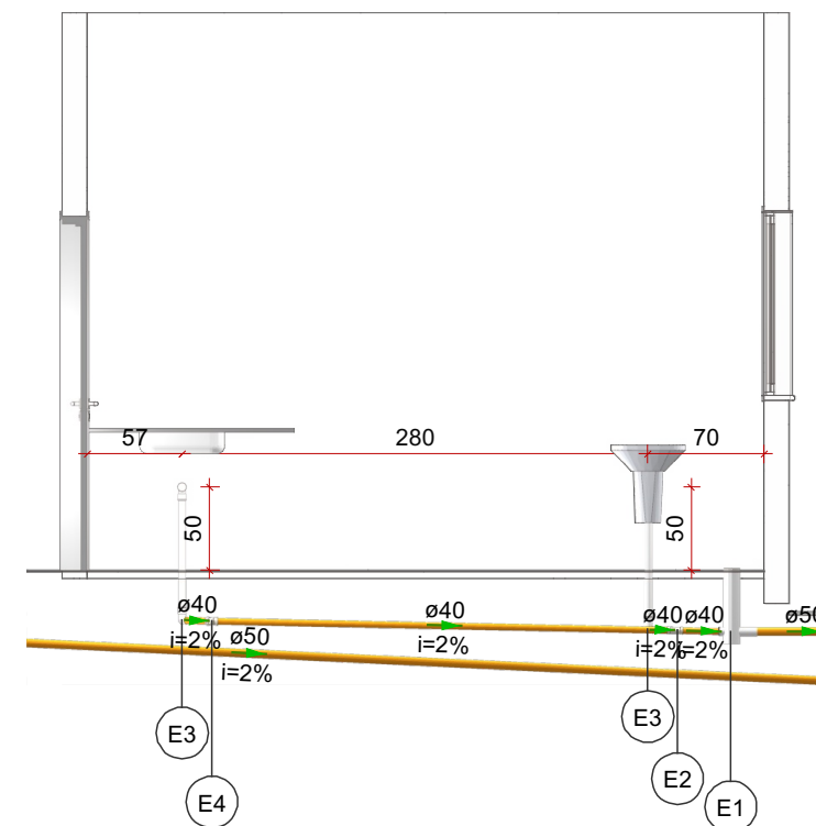
Detalhe SAN-4 Escala 1:50
