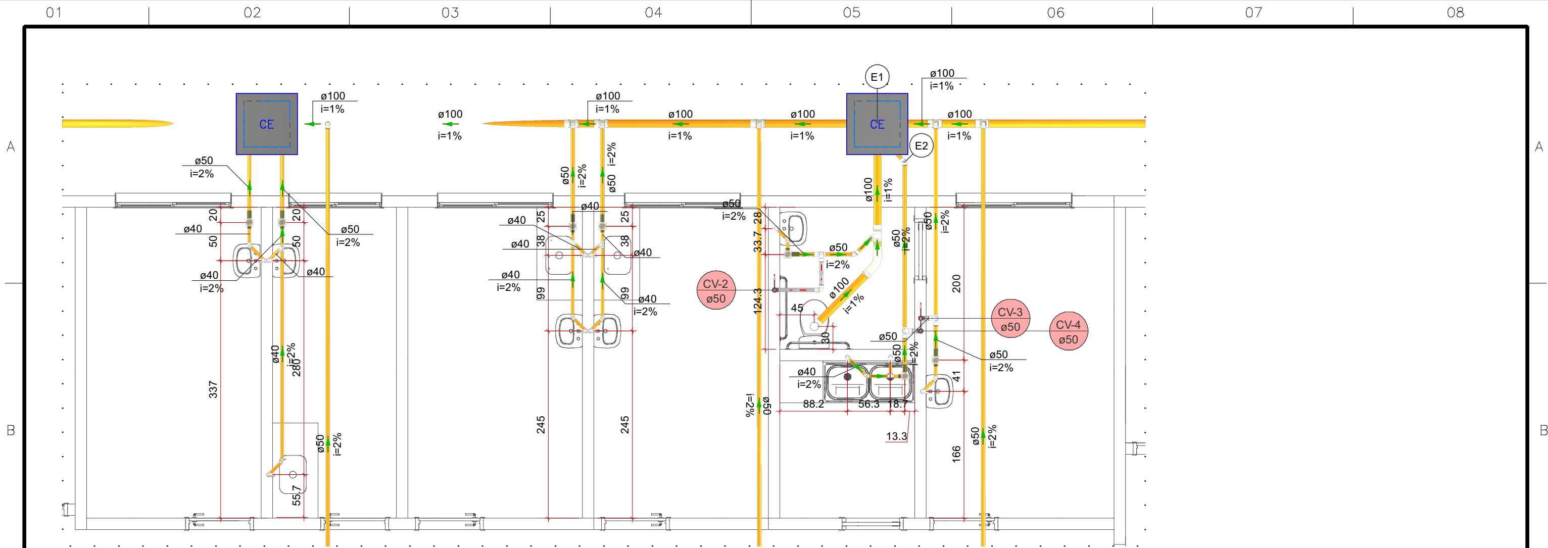
Detalhe SAN-1 Escala 1:50
