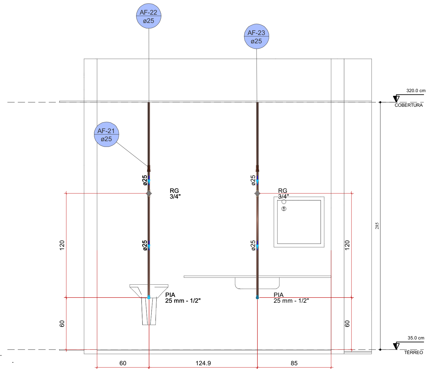
Detalhe HID-21 Escala 1:25
