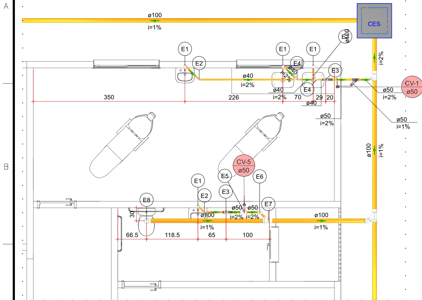
Detalhe SAN-2 Escala 1:50
