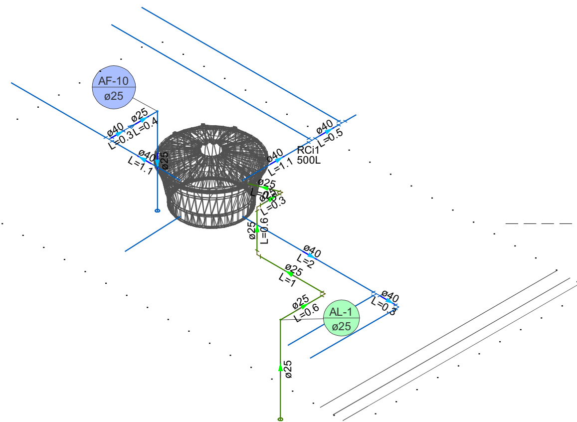
Detalhe HID-1 Escala 1:50
