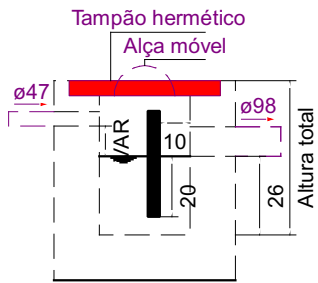
Caixa de gordura - TÉRREO Corte 1 - ESC. 1:25
