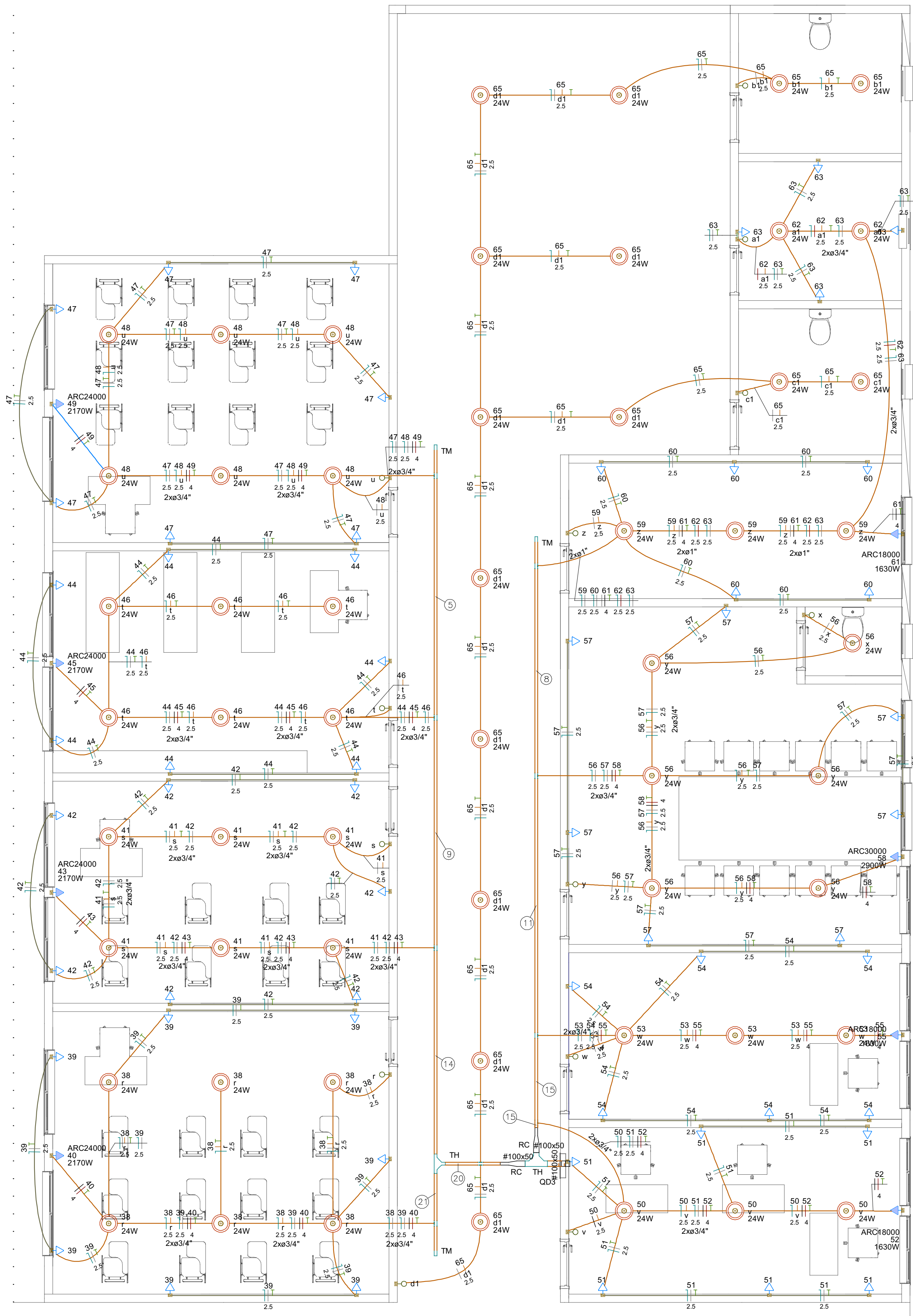
Detalhe ELE-3 Escala 1:50
